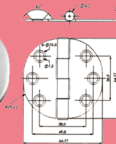
Edelstahl-Scharniere mit Abdeckung A4 NIRO AISI316
