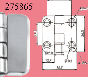
Edelstahl-Scharniere mit Abdeckung A4 NIRO AISI316
