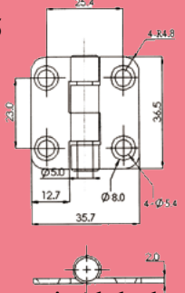
Edelstahl-Scharniere mit Abdeckung A4 NIRO AISI316
