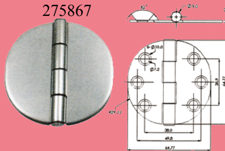
Edelstahl-Scharniere mit Abdeckung A4 NIRO AISI316
