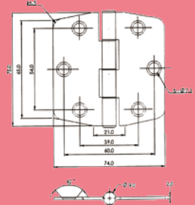
Edelstahl-Scharniere mit Abdeckung A4 NIRO AISI316
