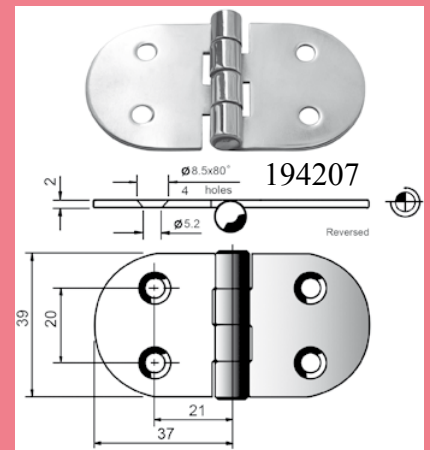
Scharnier / Edelstahl A4 NIRO AISI316
