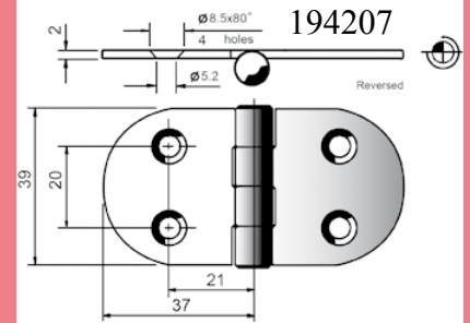
Scharnier / Edelstahl A4 NIRO AISI316
