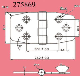
Edelstahl-Scharniere mit Abdeckung A4 NIRO AISI316
