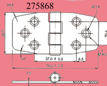
Edelstahl-Scharniere mit Abdeckung A4 NIRO AISI316
